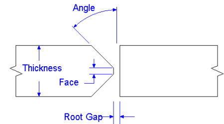
DOUBLE BEVEL
