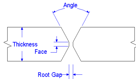
DOUBLE VEE
